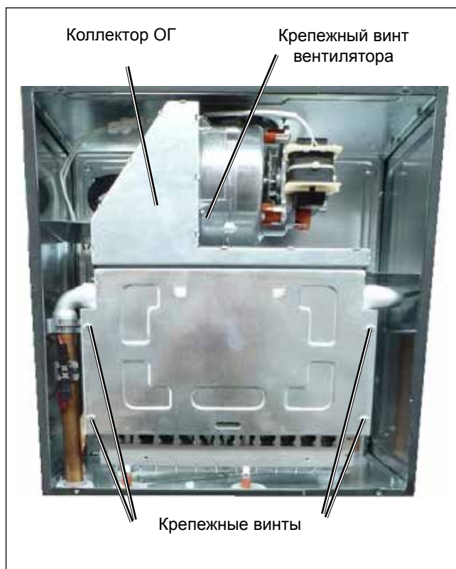
Рис. Корпус камеры сгорания
