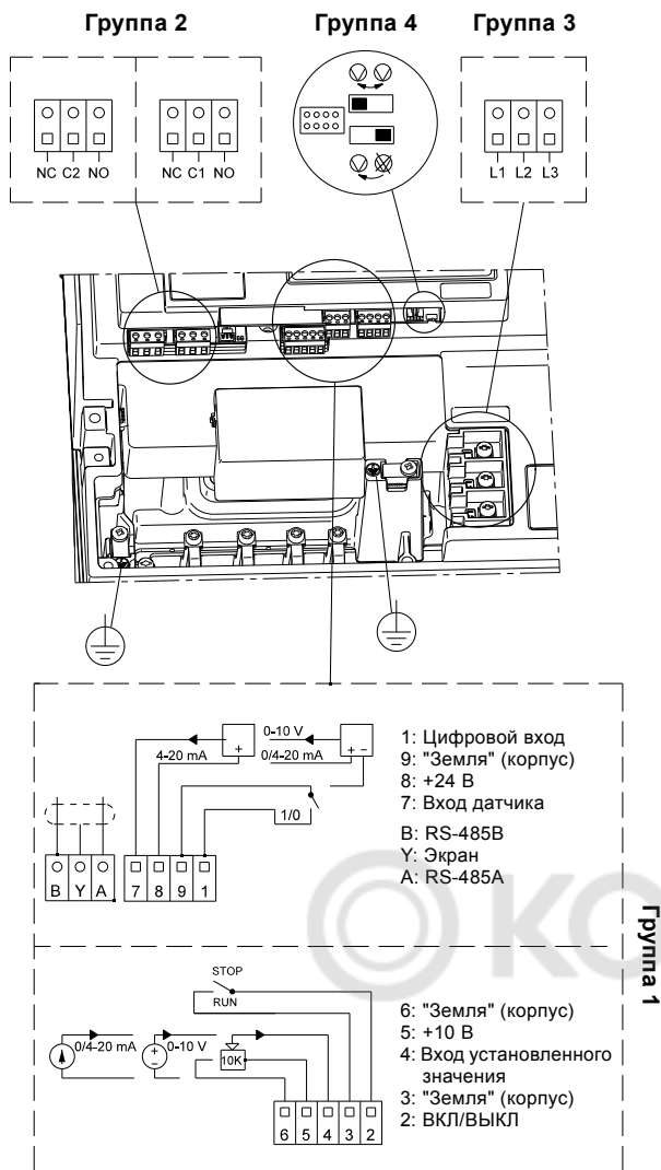
Рис. 15 Клеммы насосов TPED
