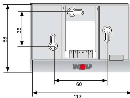
Рис. 4.5 Монтаж настенного цоколя ВМ-2 на стену с помощью винтов и дюбелей
