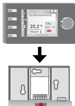
Рис. 4.6 Установка модуля управления ВМ-2 сверху в направляющие настенного модуля
