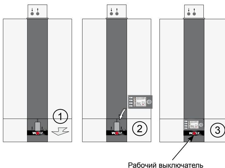
Рис. 4.1 Установка модуля управления BM-2 в CGB-2
