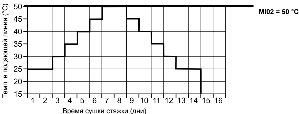
Рис. 26.1 Динамика по времени температуры в подающей линии во время сушки стяжки «Автоматика» при MI02 = 50 °C
