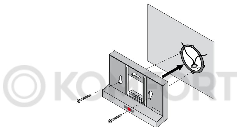
Рис. 4.4 Монтаж настенного цоколя ВМ-2 на подрозетник (предоставляется клиентом)
