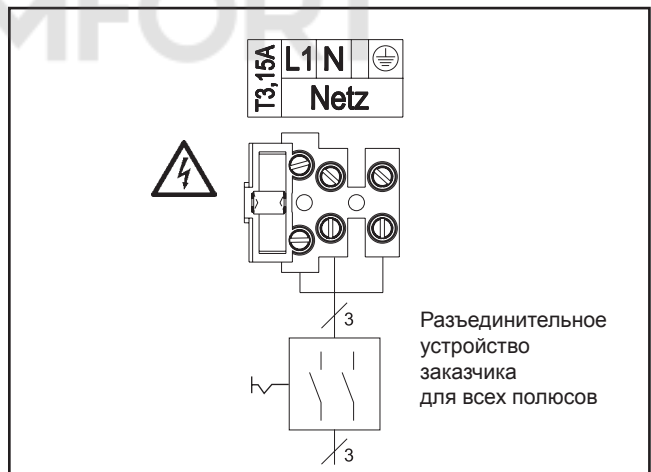
Рисунок. Электропитание
