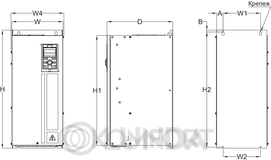
Рисунок 3.6-6. Чертеж преобразователя частоты типоразмер B6
