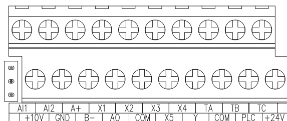
Рисунок 4.5-2. Расположение клемм цепи управления
