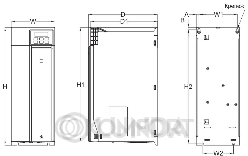
Рисунок 3.6-4. Чертеж преобразователя частоты типоразмер В4
