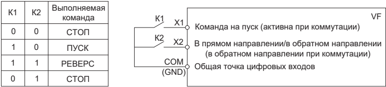
Рисунок 10.9-6. Двухпроводная схема управления 2
