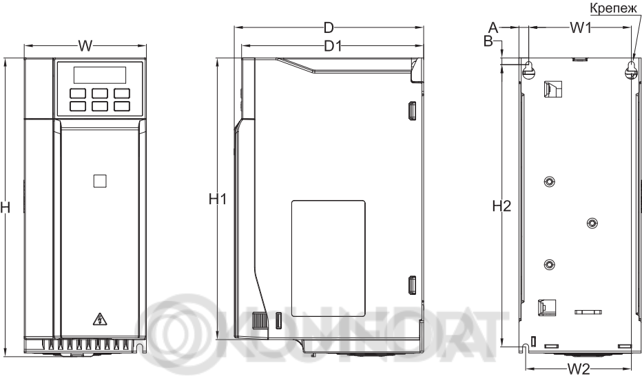
Рисунок 3.6-2. Чертеж преобразователя частоты типоразмер В2
