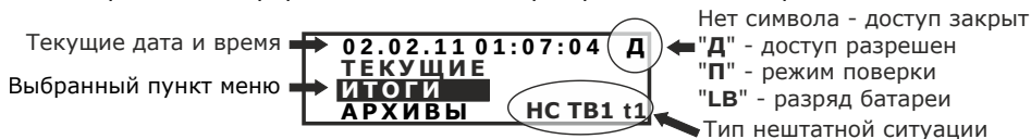
Рис. 2.5 – Отображение информации на индикаторе
