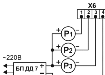
Вариант 4. Подключение ДД к ТВ7-04.1М Лайт
