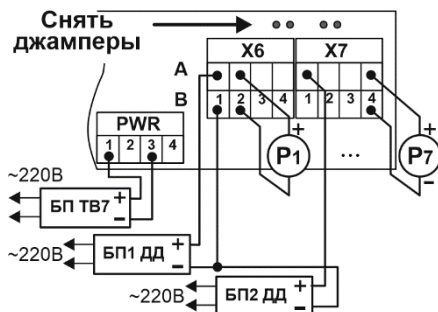
Вариант 3. Раздельное питание ТВ7 и ДД
