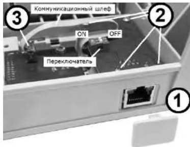
Рис. Е.1 Порядок установки адаптера
