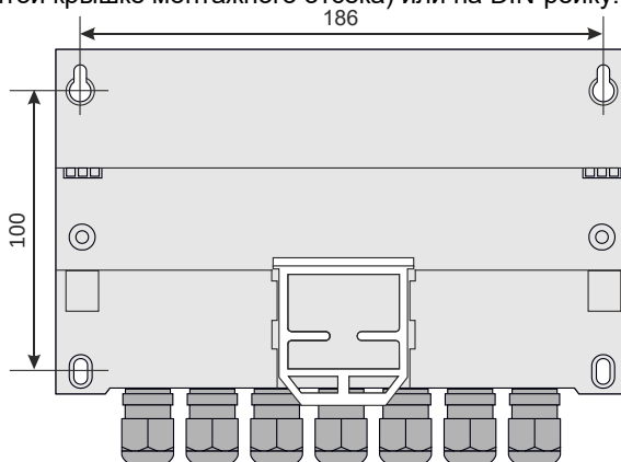
Рис. 4.1 – Схема крепления корпуса ТВ7
