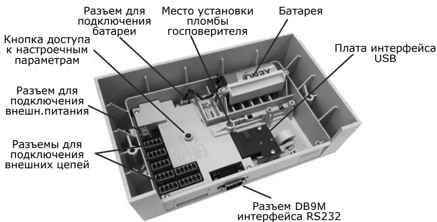
Рис. 2.3 – Вид снизу на приборный отсек TB7-04.1M Лайт
