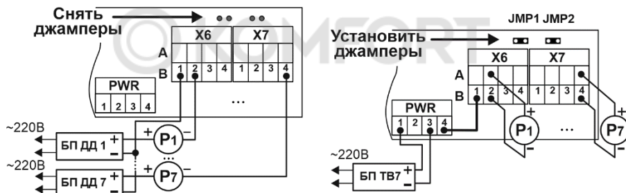
Вариант 1. Индивидуальное питание ДД
