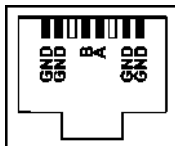
Рис. Ж.2 Цоколевка выходов разъема RJ45
