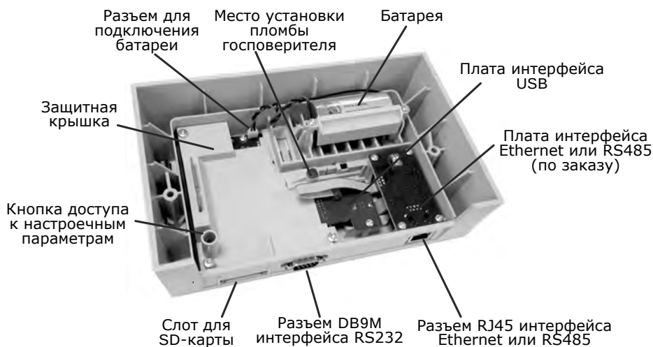
Рис. 2.2 – Вид снизу на приборный отсек TB7
