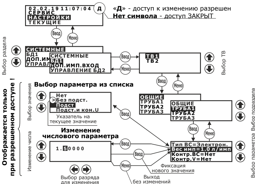
Рис. 3.1 – Пример просмотра значения параметра настройки
