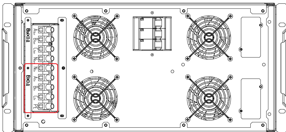
Рисунок 17б. Стабилизаторы IS3315RT и IS3320RT. Выводы «Вход N вх -А вх -В вх -С вх -РЕ»
