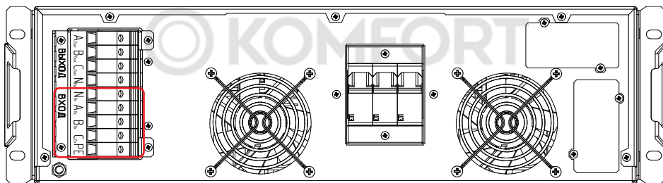
Рисунок 17а. Стабилизаторы IS3306RT, IS3308RT и IS3310RT. Выводы «Вход N вх -А вх -В вх -С вх -РЕ»
