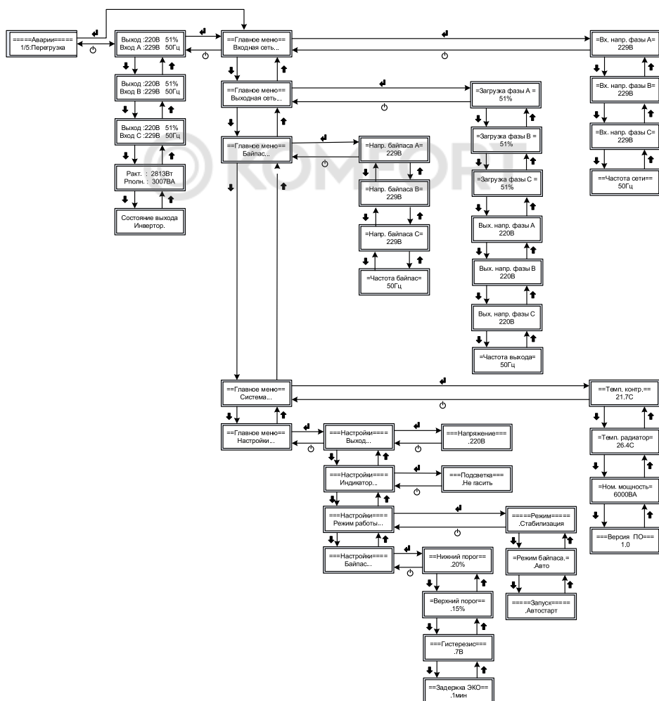
Рисунок 10. Структура меню стабилизатора
