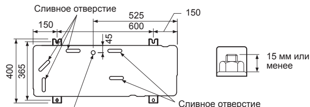
Крепежное отверстие для сливного ниппеля
