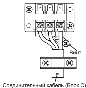
* Пример подключения (RAS-3M26U2AVG-E)
