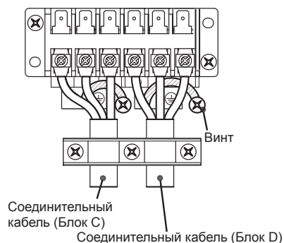
* Пример подключения (RAS-4M27U2AVG-E)
