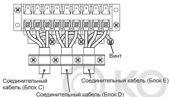
* Пример подключения (RAS-5M34U2AVG-E)
