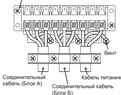
Клеммная колодка (Соединительный кабель)
