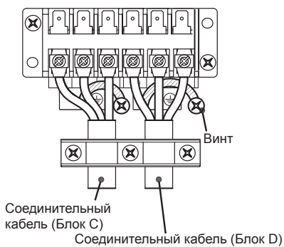
* Пример подключения (RAS-4M27U2AVG-E)
