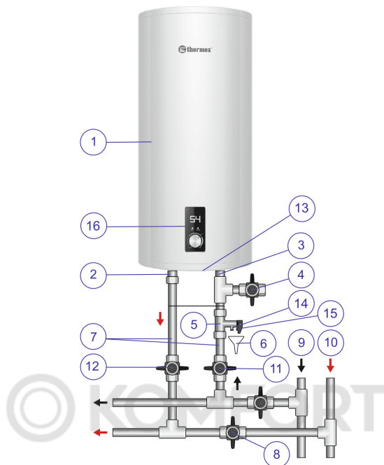
Рисунок 1. Схема подключения ЭВН к водопроводу
