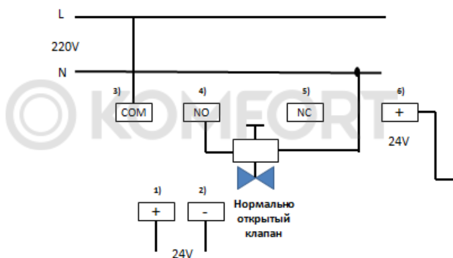
Схема №1. Подключение сигнализатора с нормально-открытым клапаном
