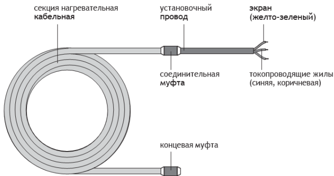
Рис. 1 - Конструкция секции нагревательной кабельной Freezstop Inside Dachа
