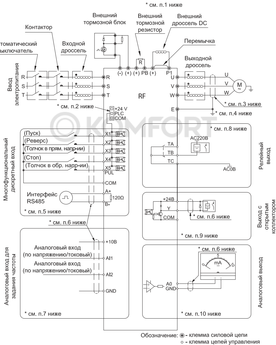
Рисунок 4.5-1. Схема внешних подключений
