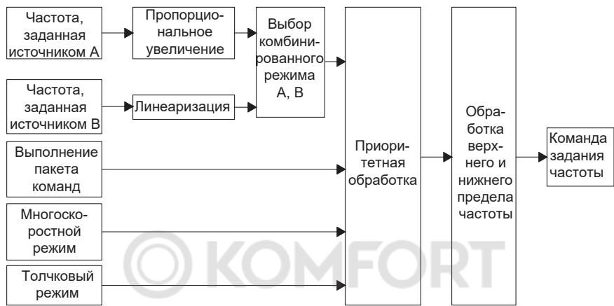
Рисунок 10.5-1. Схема задания частоты
