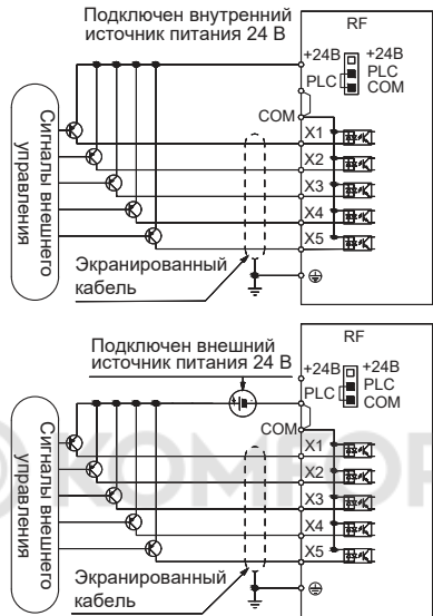
Рисунок 4.7-1. Способ подключения логики PNP
