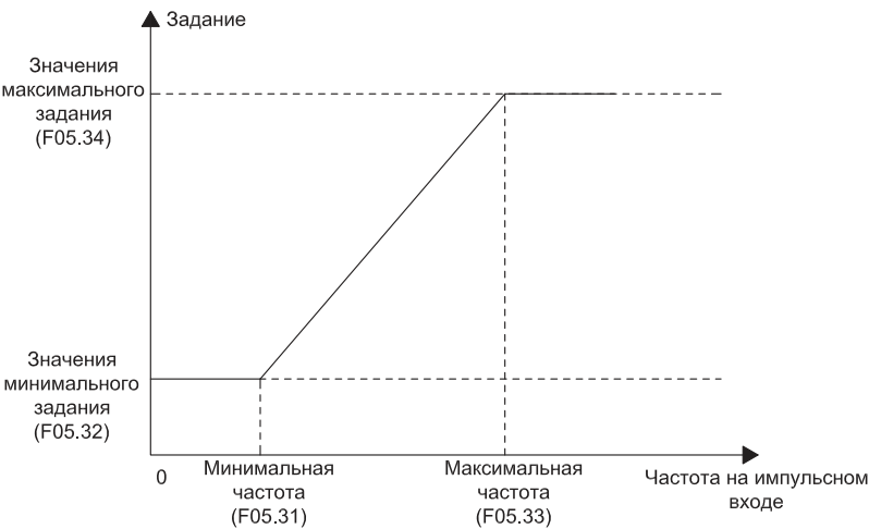
Рисунок 10.9-9. Обработка частоты сигнала, поступающего на импульсный вход
