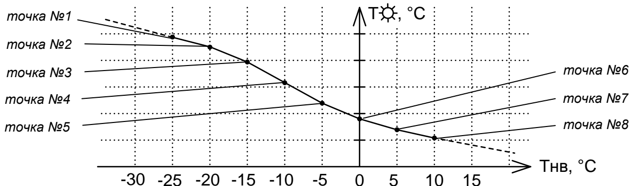
Рисунок 7 - Температурный график
