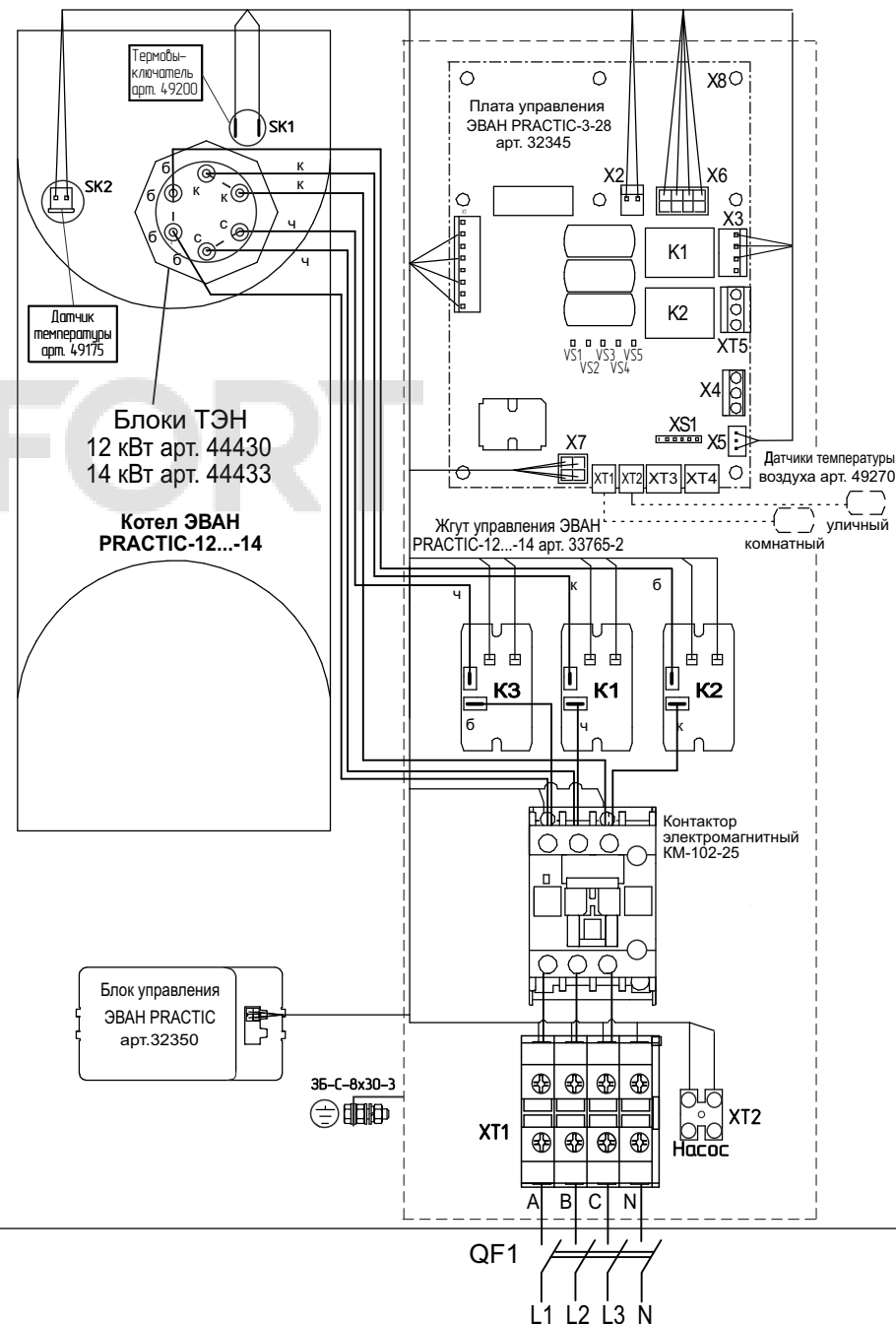
Рисунок 20. Схема подключения ЭВАН PRACTIC-12...-14.
