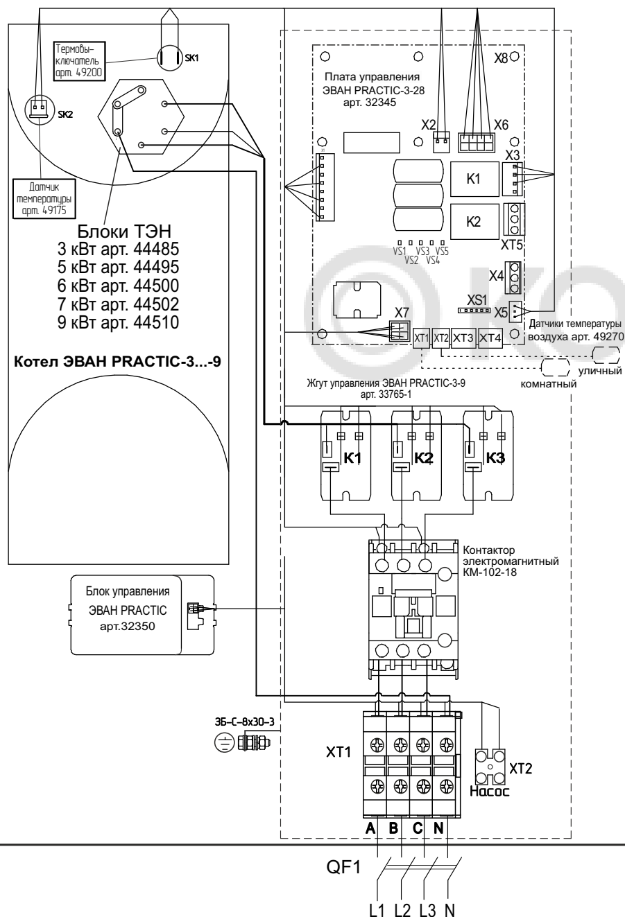
Рисунок 19. Схема подключения ЭВАН PRACTIC-3...-9 к сети 380В.
