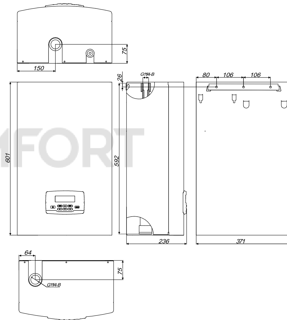
Рисунок 16. Габаритные и присоединительные размеры прибора ЭВАН PRACTIC -3 ... -28
