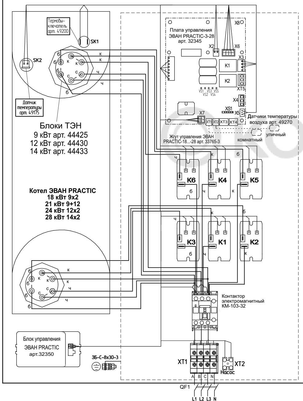
Рисунок 21. Схема подключения ЭВАН PRACTIC-18...-28.
