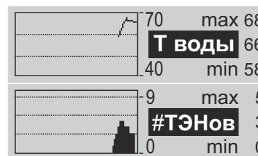
Рисунок 10. Графики динамики числа включенных ТЭНов и температуры теплоносителя
