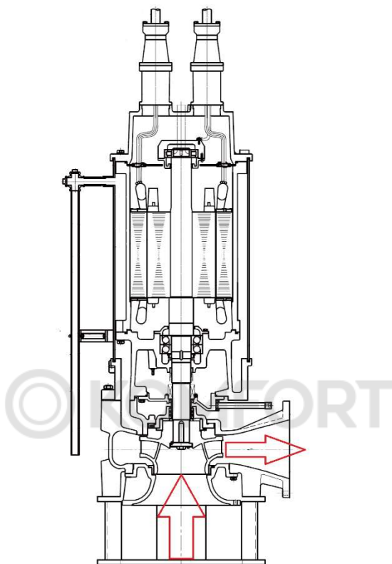
Рис. 8 Схема расположения патрубков насоса
