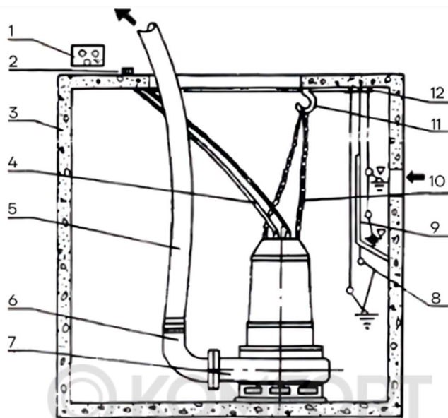
Рис. 6 Переносная установка
