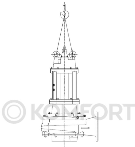
Рис. 2 Схема строповки насоса без тары
