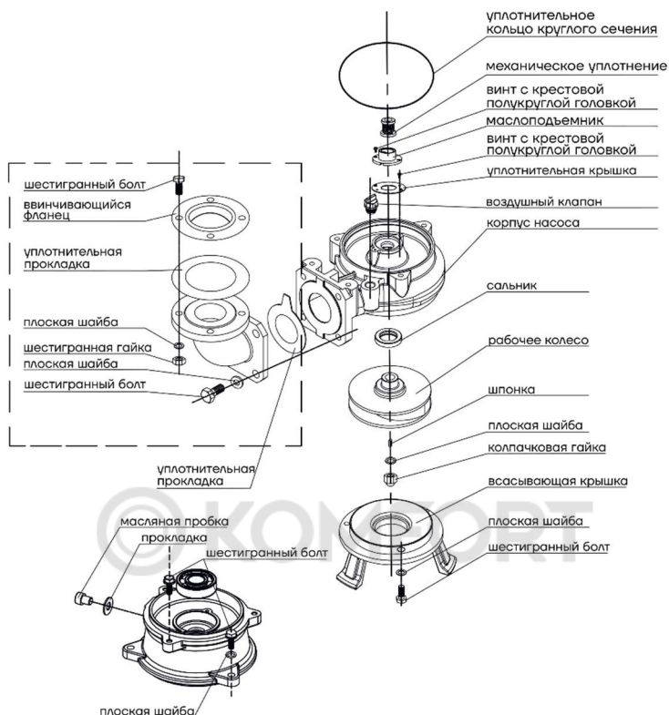
Рис. 17 Типовая взрывная схема насосов серии WQ
