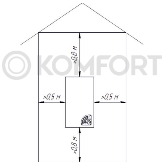
Рисунок 3. Схема установки
