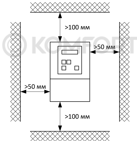
Рисунок 3 – Установка ПЧ
