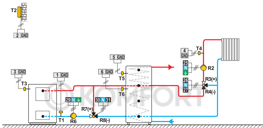
Схема 415b (W20) - ТТ котел, бак-теплоаккумулятор, смесительный контур, бойлер ГВС
