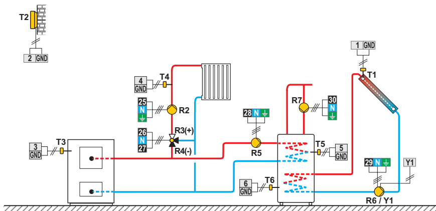
Схема 404с (W10, W20) - ТТ котел, смесительный контур, бойлер ГВС, солнечный коллектор
