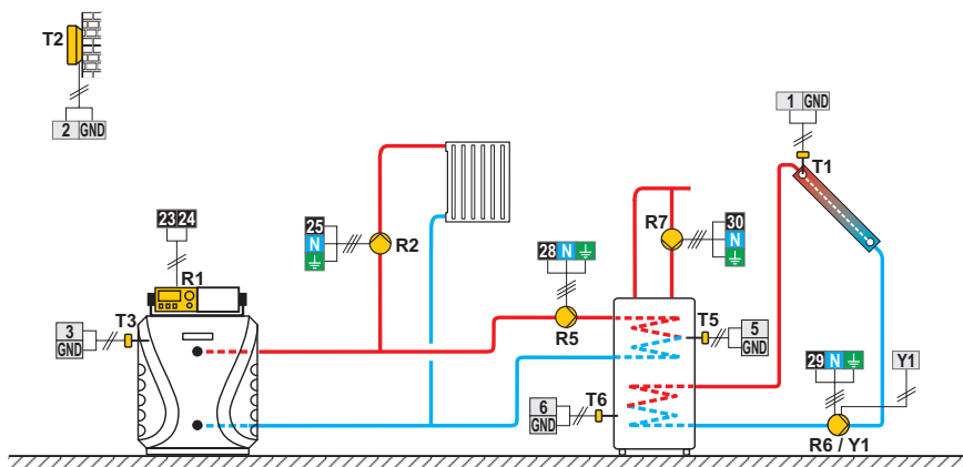
Схема 405 (W10, W20) - ЖТ котел, прямой контур, бойлер ГВС, солнечный коллектор
