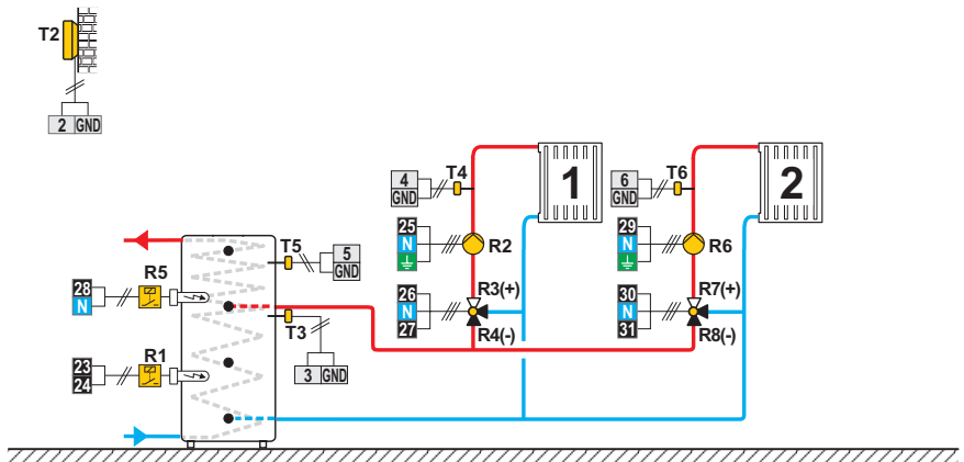
Схема 423d (W20) - Схема расширения — бак-теплоаккумулятор с встроенным бойлером ГВС, 2 смесительных контура
