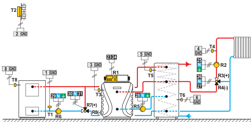
Схема 415с (W20) - ЖТ котел, ТТ котел, бак-теплоаккумулятор с встроенным бойлером ГВС, смесительный контур
