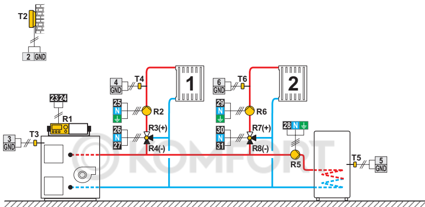
Схема 423g (W20) - Комбинированный котел (ЖТ/ТТ), 2 смесительных контура, бойлер ГВС
