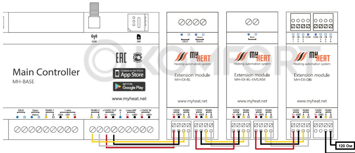
Рис.3. Схема подключения модулей в шлейф
