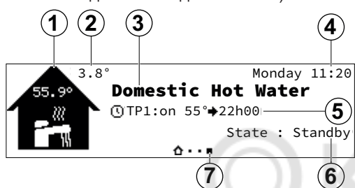
Рис.8 Основная индикация для страницы ГВС (только при подключении датчика ГВС)
