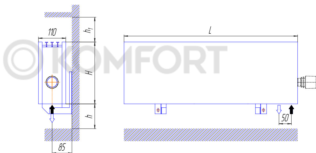
Рис. 1 Конвектор «Эlegant». Напольное исполнение: а) – на ножках фиксированной высоты; б) – на регулируемых ножках.
