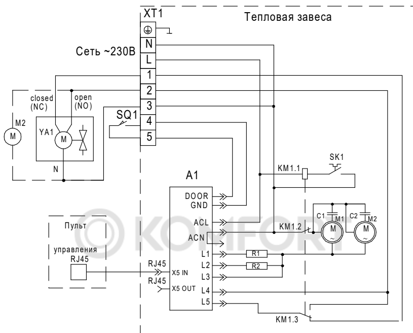
Рисунок 18. Схема электрическая принципиальная подключения завесы KVC-D20W50-11
