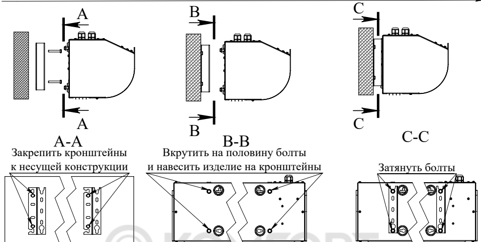
Рисунок 13. Схема крепления завесы горизонтально над проемом к стене с помощью кронштейнов.
