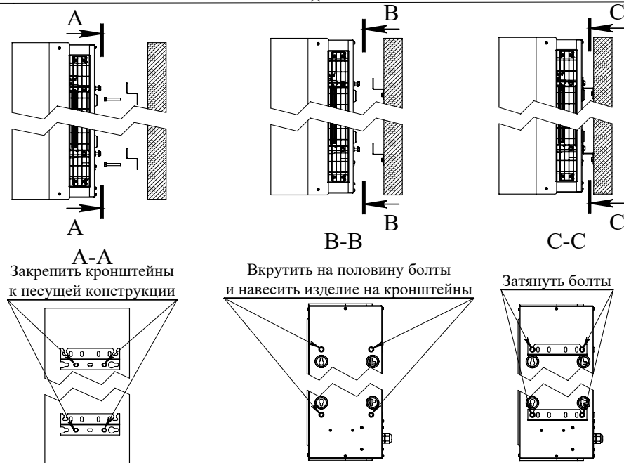
Рисунок 14. Схема крепления завесы вертикально к стене с помощью кронштейнов.
