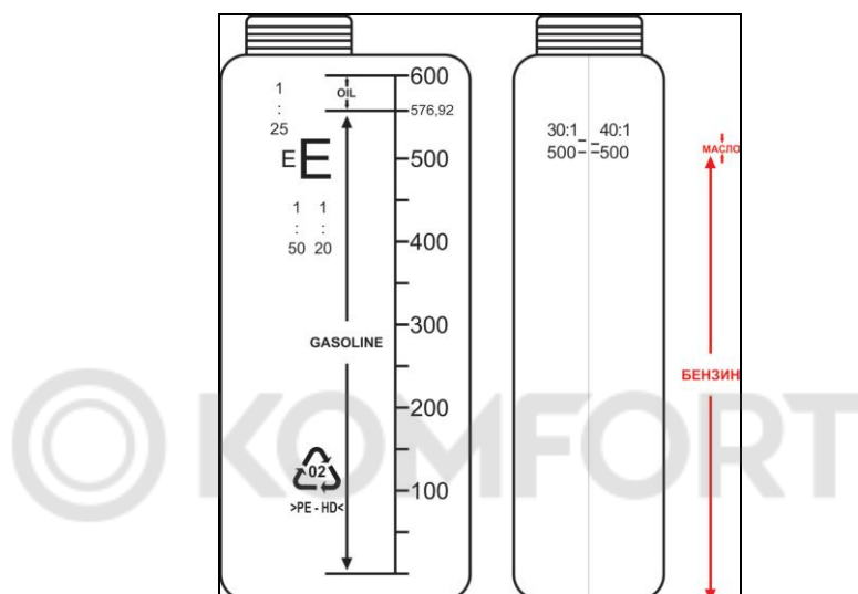
Рис. 11. Емкость для приготовления топливной смеси
