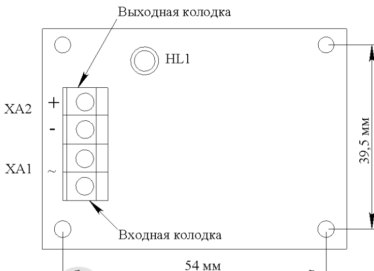
Рисунок – Преобразователь напряжения ПН-24АС/12-1,0
