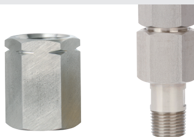
Рис. слева: Соединительный переходник, накидная гайка с левой/правой резьбой, G ½ / G ½ LH
