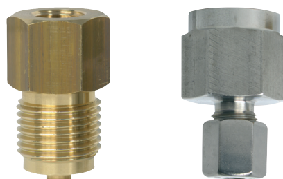
Рис. слева: Переходник с наружной резьбы на внутреннюю резьбу, G ½ / G ¼ В
