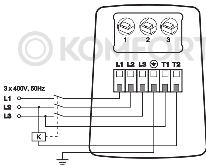
Рис.4. Схема подключения трехфазного насоса.
