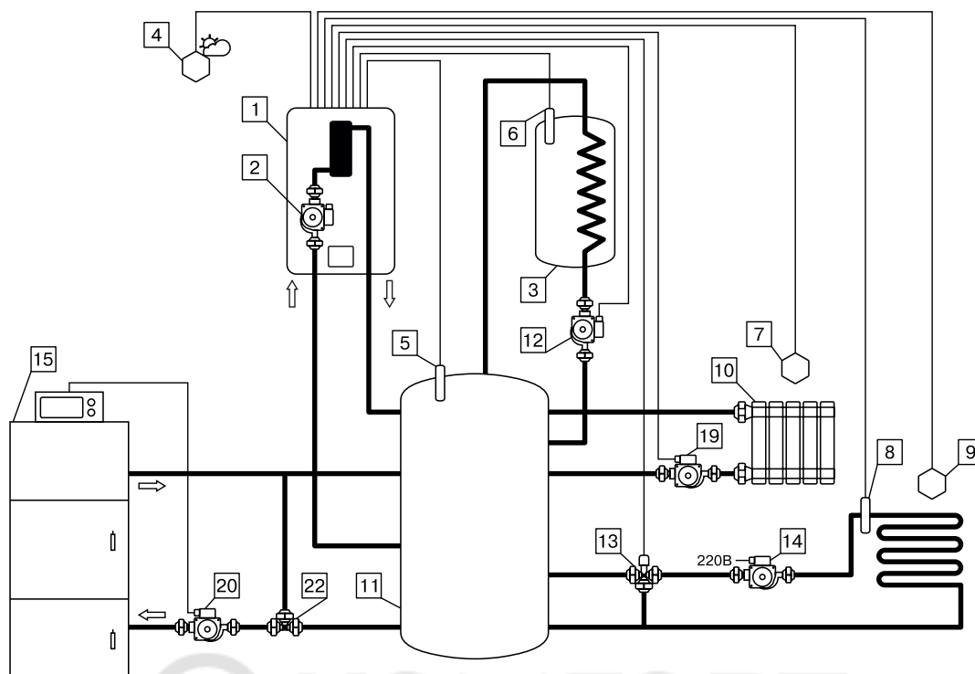
Схема 4. Совместная работа основного котла с блоком управления с электродом с активированной функцией «Бак аккумулятор», насосом 2 в режиме ГВС или отопление, насосом 3 в режиме отопление и клапаном в режиме работы «Смешивающий».
