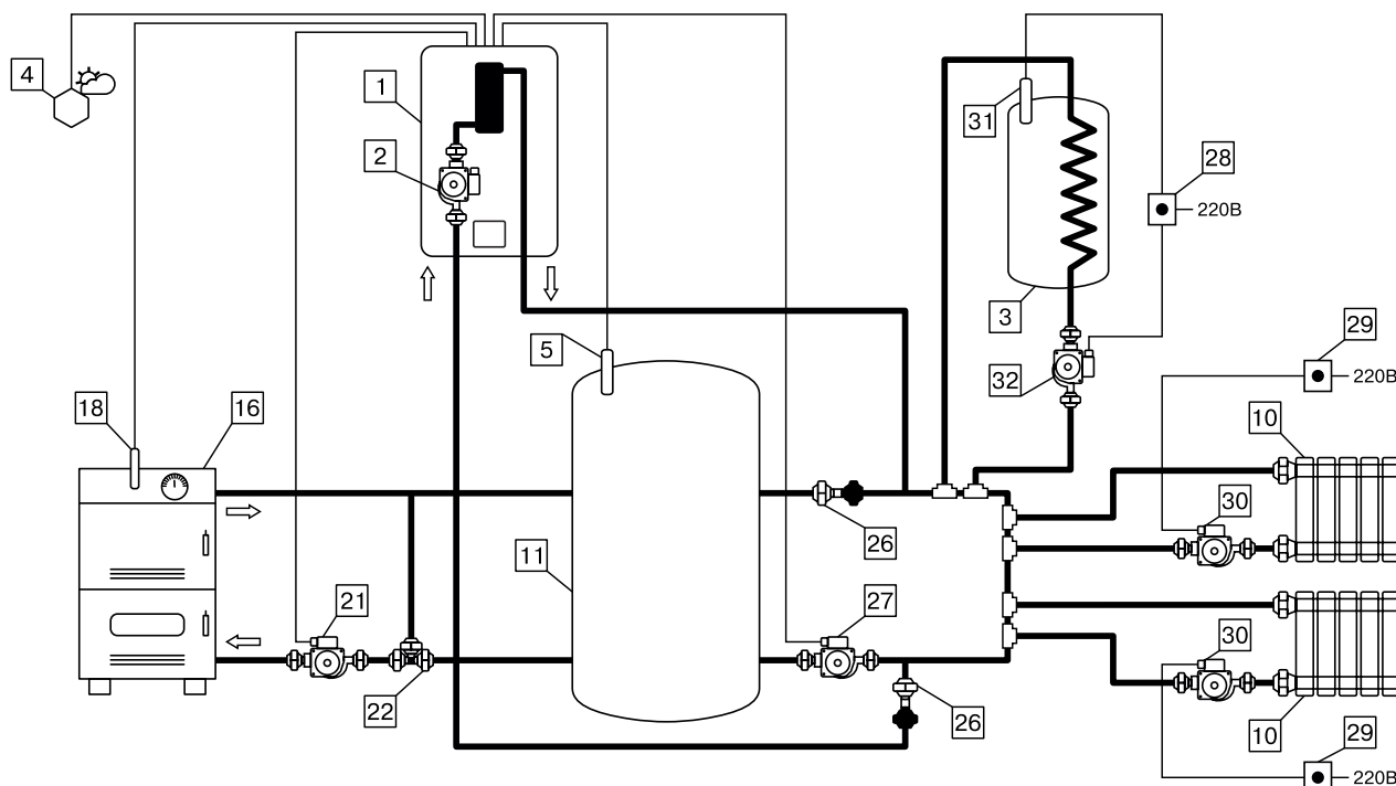
Схема 4.1. Совместная работа основного котла с электродом в режиме вспомогательный с активированной функцией «Бак аккумулятор» и насосом 2 в режиме «насос за баком аккумулятора».
