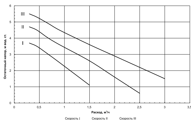
Рис.1.2 Остаточный напор для циркуляционного насоса 25/70 (Для котлов МК-S 24-36 кВт)
