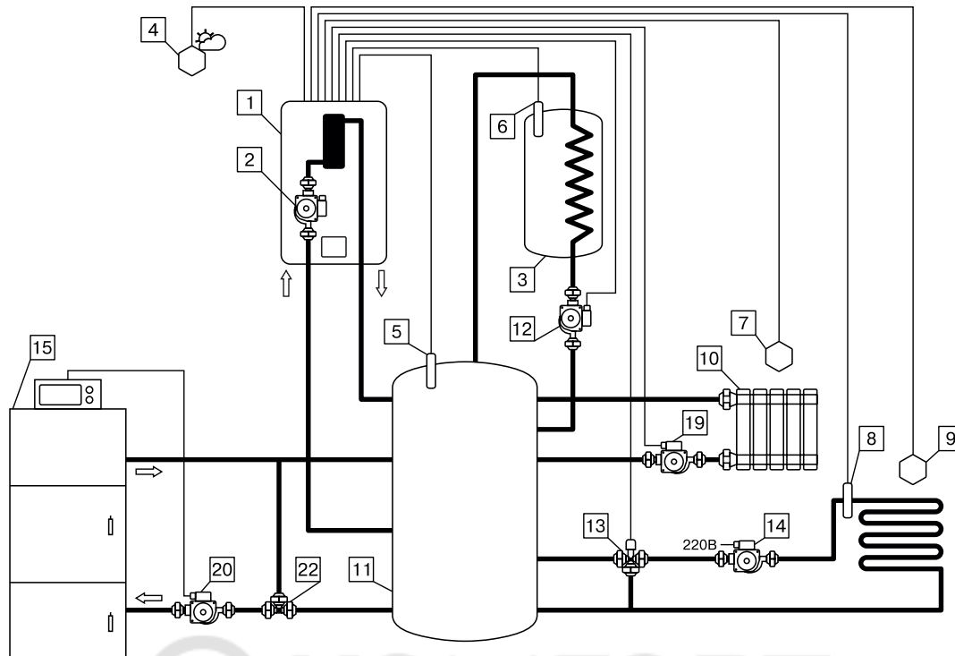
Схема 4. Совместная работа основного котла с блоком управления с электродом с активированной функцией «Бак аккумулятор», насосом 2 в режиме ГВС или отопление, насосом 3 в режиме отопление и клапаном в режиме работы «Смешивающий».
