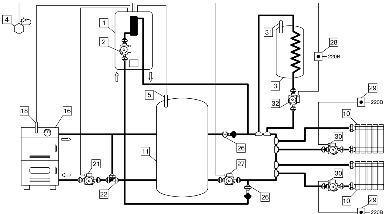
Схема 4.1. Совместная работа основного котла с электродом в режиме вспомогательный с активированной функцией «Бак аккумулятор» и насосом 2 в режиме «насос за баком аккумулятора».
