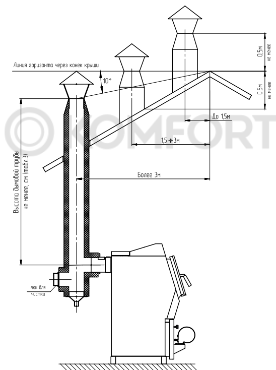
Рис.5 Варианты установки дымовой трубы
