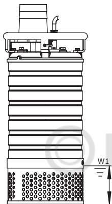
Рис. 4 Мин. размеры прямка
