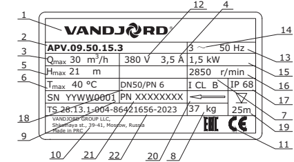
Рис. 2 Фирменная табличка насосов
