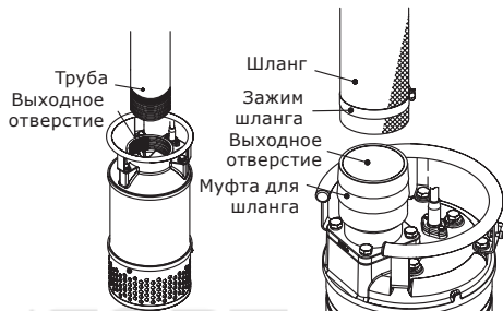
Рис. 6 Стационарная установка
