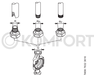
Рис. 21 Резьба G и резьба R
