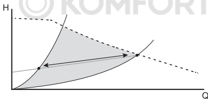
12-сур. Пропорционалдық қысым режимінде қысық пропорционалдық қысымның мысалы
