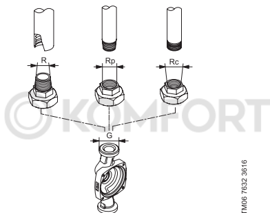
21-сур. G резьбасы және R резьбасы
