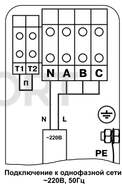
Рис.4 Схема подключения котла к однофазной сети
