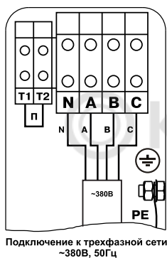
Рис.3 Схема подключения котла к трехфазной сети
