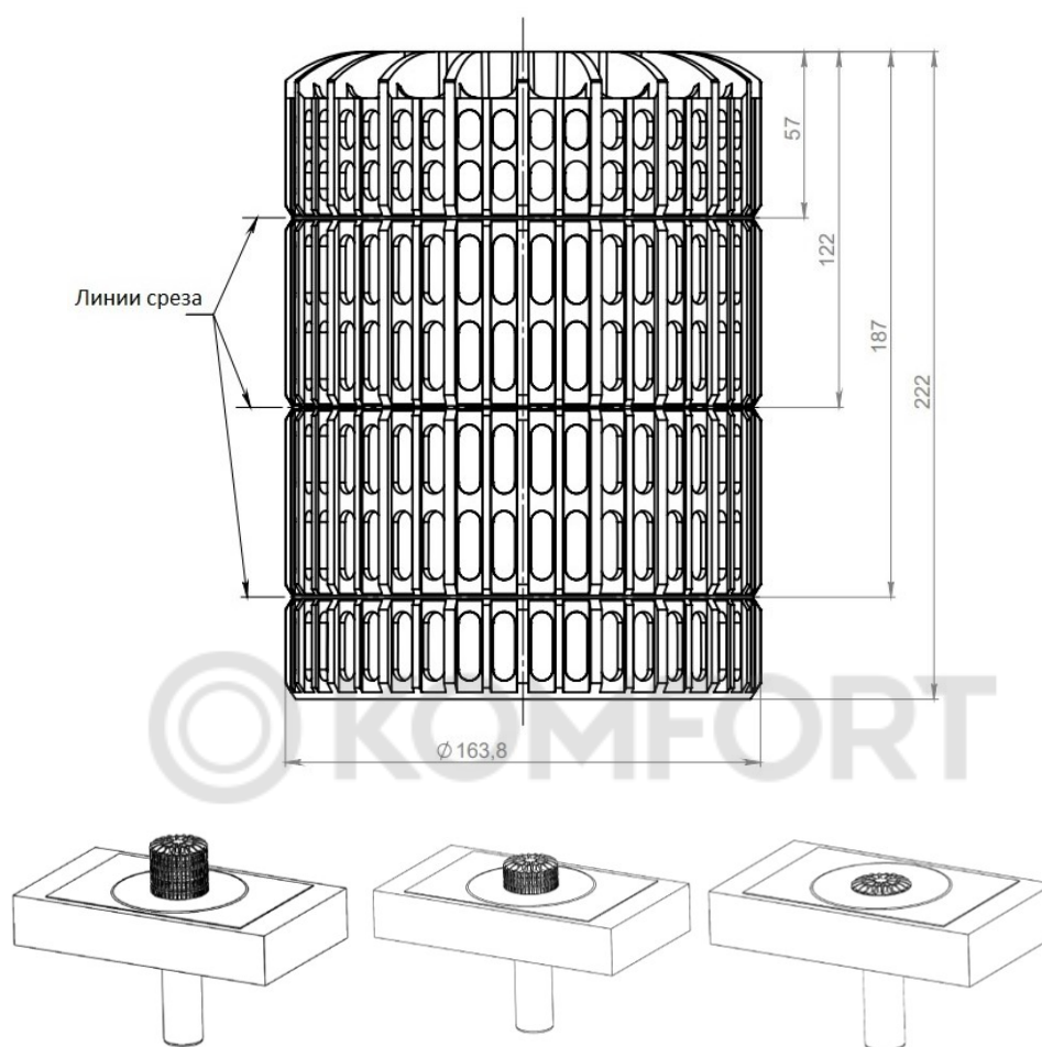
Рис. 3. Схема листоуловителя
