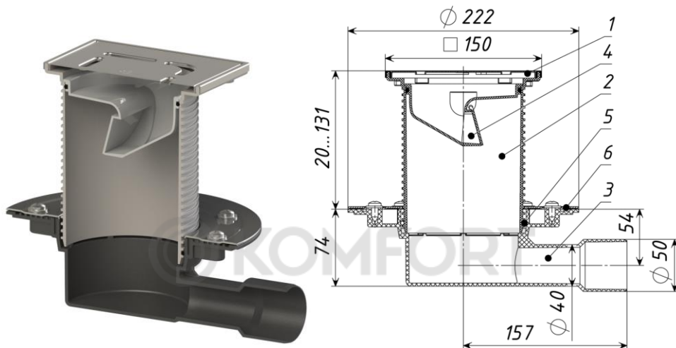
Рис. 1 ТП-510.1N-3000 Трап с незамерзающим запахозапирающим устройством
