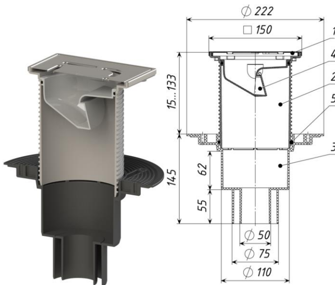
Рис. 1 ТП-310N-3000 Трап с незамерзающим запахозапирающим устройством
