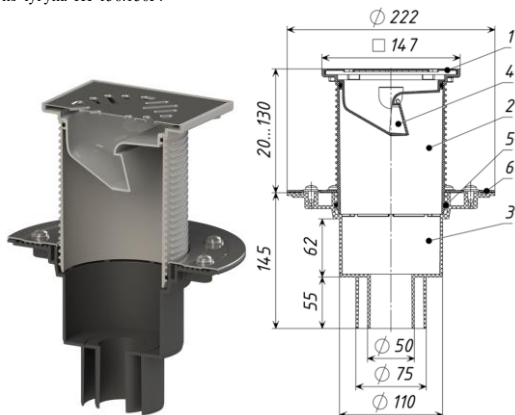
Рис. 1 ТП-310.1N Трап с незамерзающим запаховзапирающим устройством
