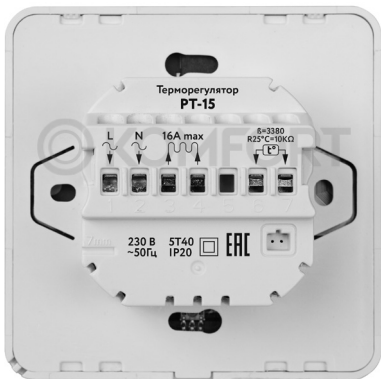
Рис. 2 Вид сзади терморегулятора PT-15
