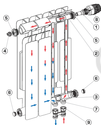
Рис. 1. Устройство радиатора
