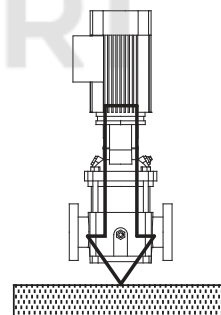
Рис. 4 Правильный монтаж
