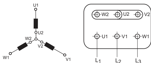
Рис. 11 Соединение звездой
