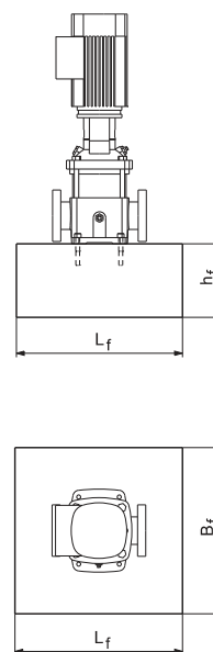
Рис. 4 Правильный монтаж
