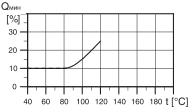
Рис. 20 Минимальная подача
