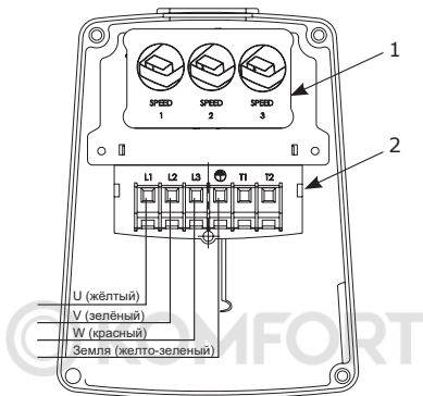
Рис. 6 Модуль переключения частоты вращения
