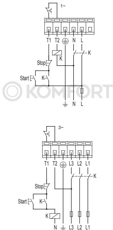
Рис. 8 Схема подключения при использовании внешнего электромагнитного пускателя ВКЛ/ВЫКЛ
