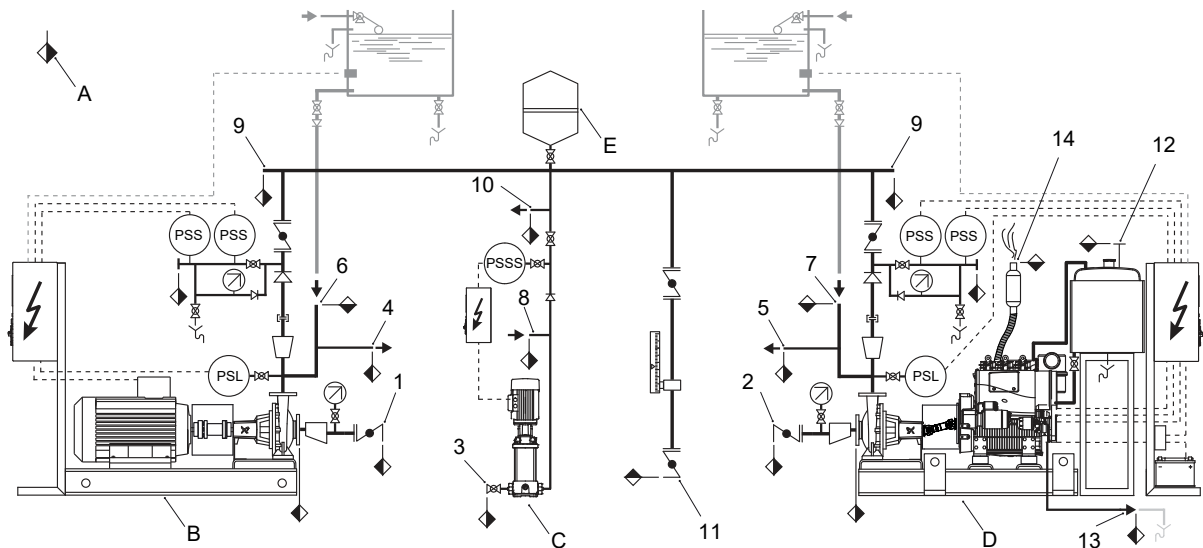
Принципиальная схема
