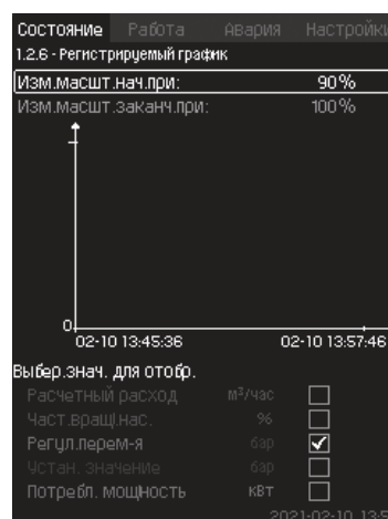
Рис. 19 Регистрируемый график
