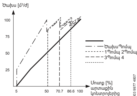
Նկար 29 Կարգավորման բնութագիր MPC-E-ի համար անջատված կոնտուրում
