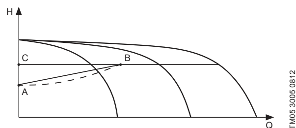
Рис. 53 Пропорц. давление
