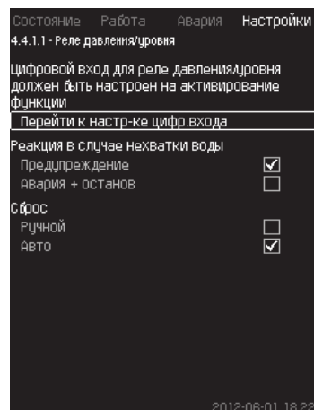
Рис. 105 Реле давления/уровня
