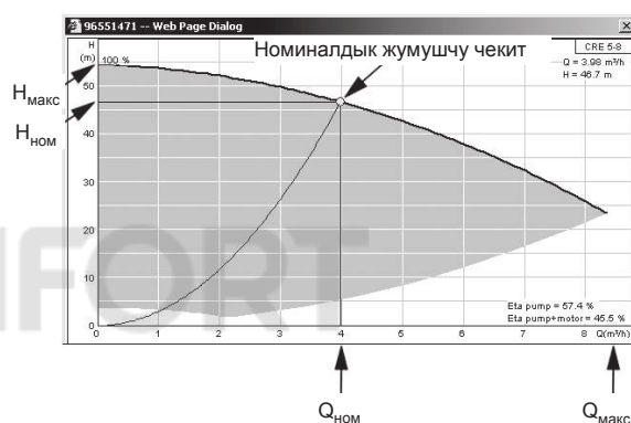
93-сур. Q_{ном} көрсөткүч, H_{ном} , H_{макс} жана Q_{макс}
