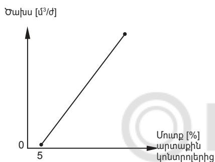
Նկար 28 Անջատված կոնտուրի համար կարգավորման բնութագիր
