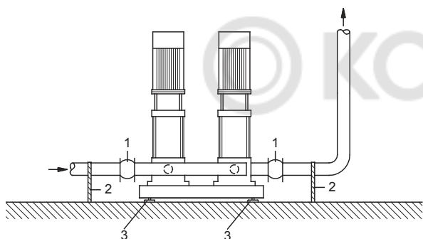
6-сур. Титирөөгө койгучтардын, түтүктөр өчүүн тирөөчтөрдүн жана титирөө тирөөчтөрүнүн абалы
