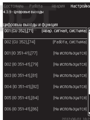
Рис. 83 Цифровые выходы
