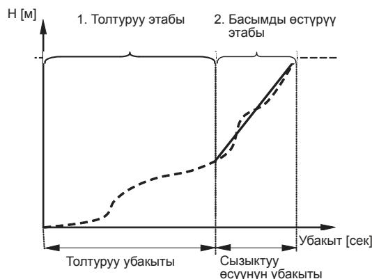
76-сур. Толтуруунун жана басымдын өсүү этаптары
