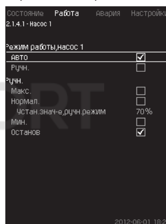
Рис. 34 Насос 1 - 6
