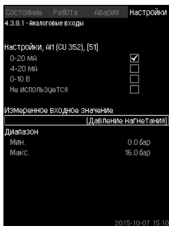
Рис. 75 Аналоговые входы
