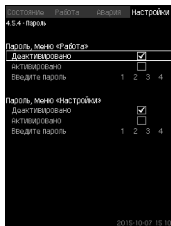
Рис. 113 Пароль
