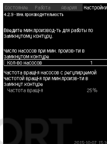
Рис. 61 Мин. производительность
