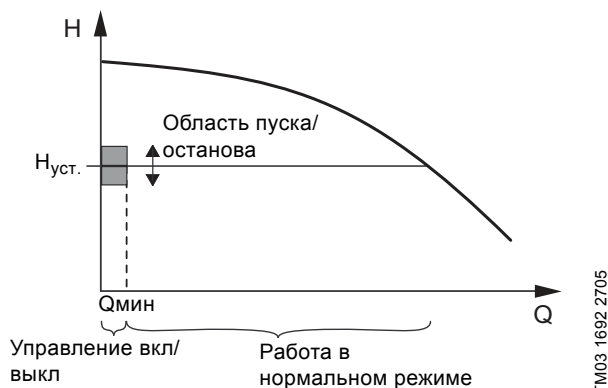
Рис. 65 Область пуска/останова
