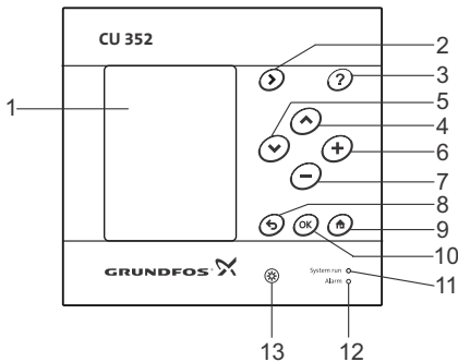
Рис. 4 Панель управления
