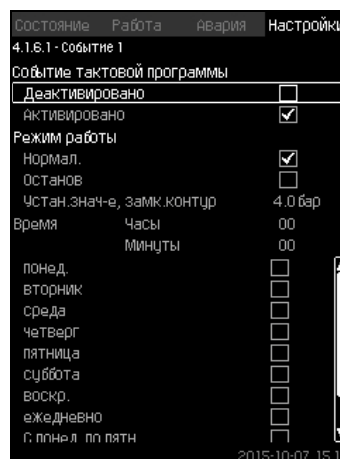
Рис. 46 Событие 1
