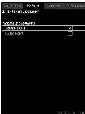
Рис. 19 Режим управления
