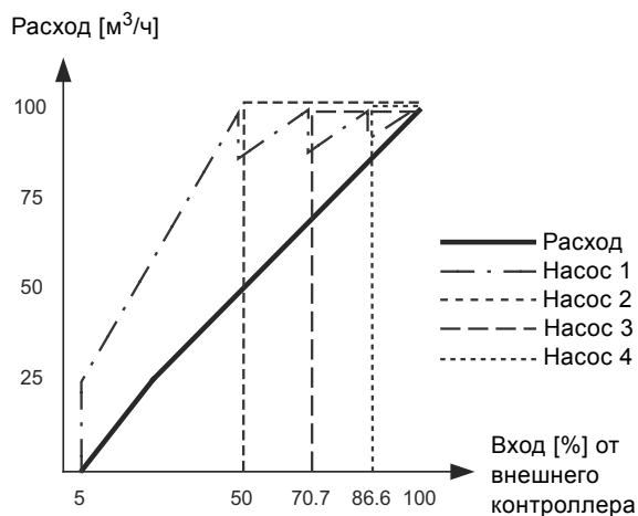
Рис. 25 Регулировочная характеристика для MPC-F в разомкнутом контуре
