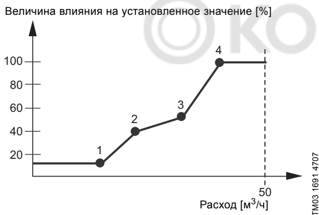
Рис. 43 Соотношение между влиянием на установленное значение и расходом
