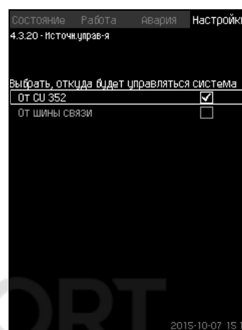
Рис. 90 Источн.управ-я
