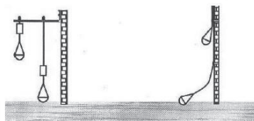
Рис. 2 Монтаж поплавкового выключателя MS M2
