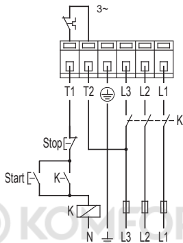
Рис. 8 Схема подключения при использовании внешнего электромагнитного пускателя ВКЛ/ВЫКЛ
