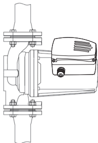
Рис. 2 Допустимое расположение вала насоса
