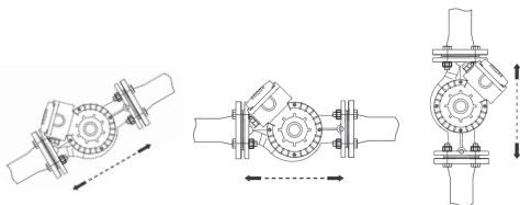
Рис. 4 Расположение клеммной коробки
