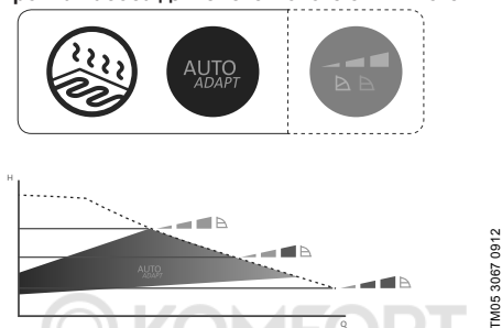
Рис. 20 Выбор настроек насоса в соответствии с типом системы. Заводская настройка: AUTO_{ADAPT} .
