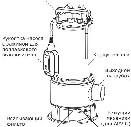
Рис. 4 Конструкция насосов APV.40B/45B/50B V/G
