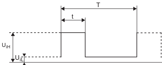
Նկար 15 LhU ազդանշանի ցուցադրություն
