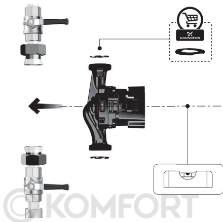
4-сур. Сорғыны құрастыру
