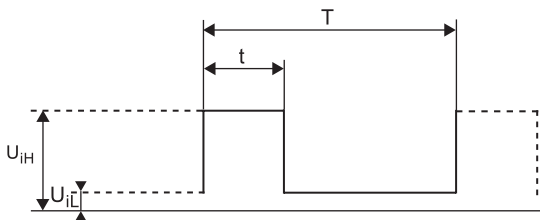
15-сур. ЕИМ сигналдың суретпен көрсетілуі
