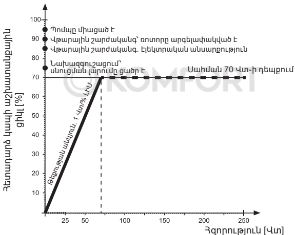
Նկար 17 Հետադարձ կապի ԼԻՄ ազդանշանի պրոֆիլը
