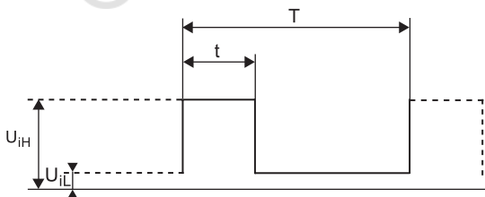
Рис. 15 Иллюстрация ШИМ сигнала
