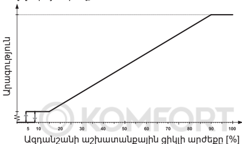
Նկար 16 ԼիՄ մուտքային ազդանշանի «C» պրոֆիլը ALPHA SOLAR-ում
