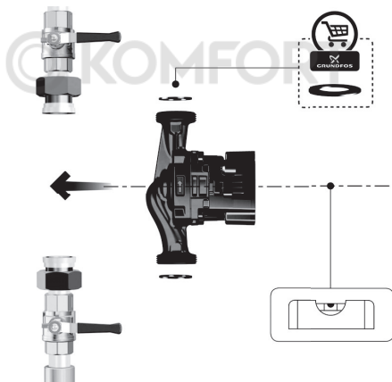
Նկար 4 Պոմպի տեղադրումը
