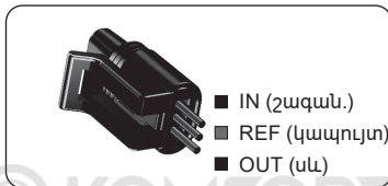
Նկար 11 Mini Superseal հարակցիչ
