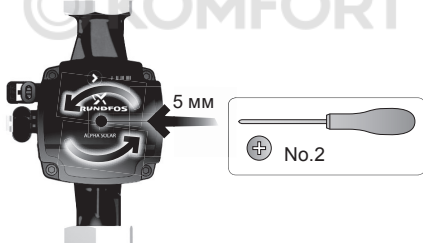
Рис. 19 Разблокировка вала насоса
